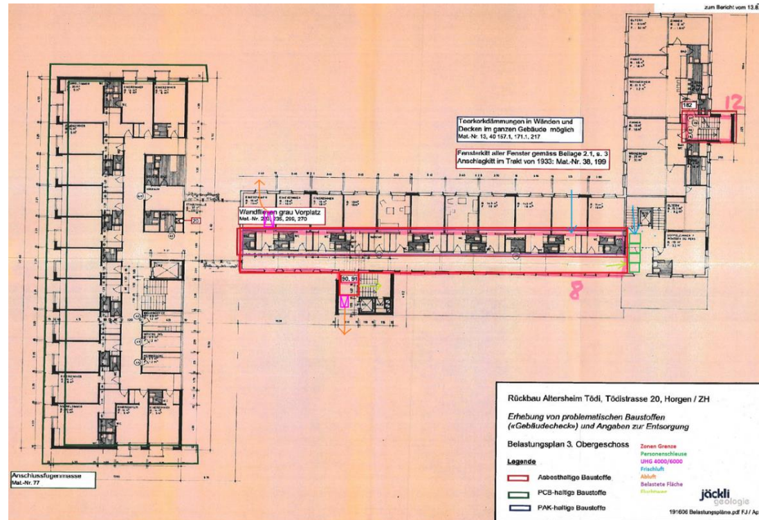
Zonenplan 3. OG
