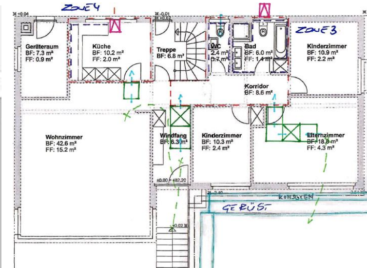
Beispiel Zonenplan EG
