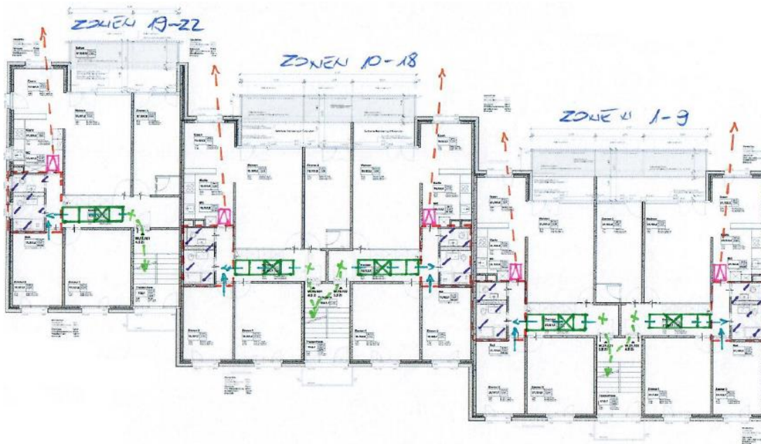
Zonenplan
