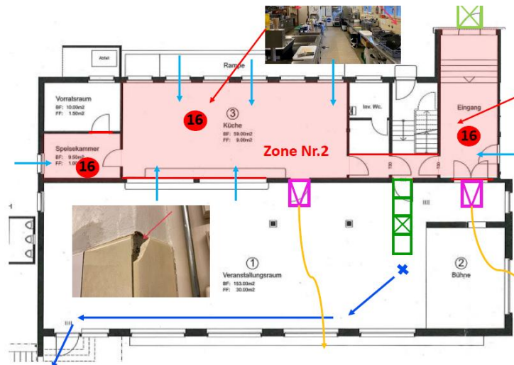
Zonenplan Erdgeschoss
