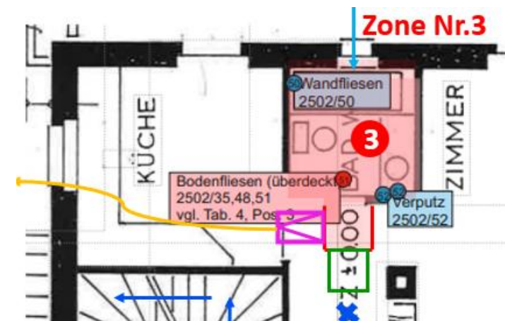
Beispiel Zonenplan
