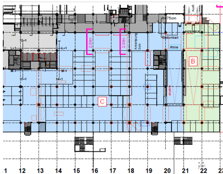
Beispiel Zonenplan
