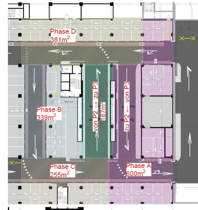
Beispiel Zonenplan
