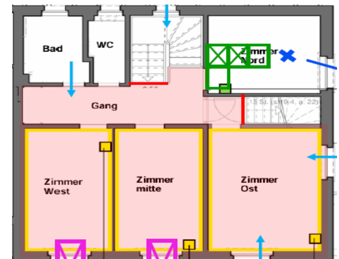
Beispiel Zonenplan Siedlung Grabenacker
